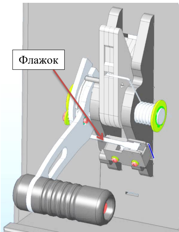
Рисунок 8 - Регулировка микропереключателя подгибкой флажка
