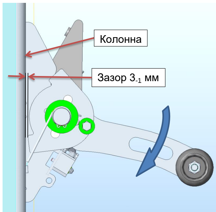
Рисунок 7 - Положение ручки управления стопорами при срабатывании микропереключателя
