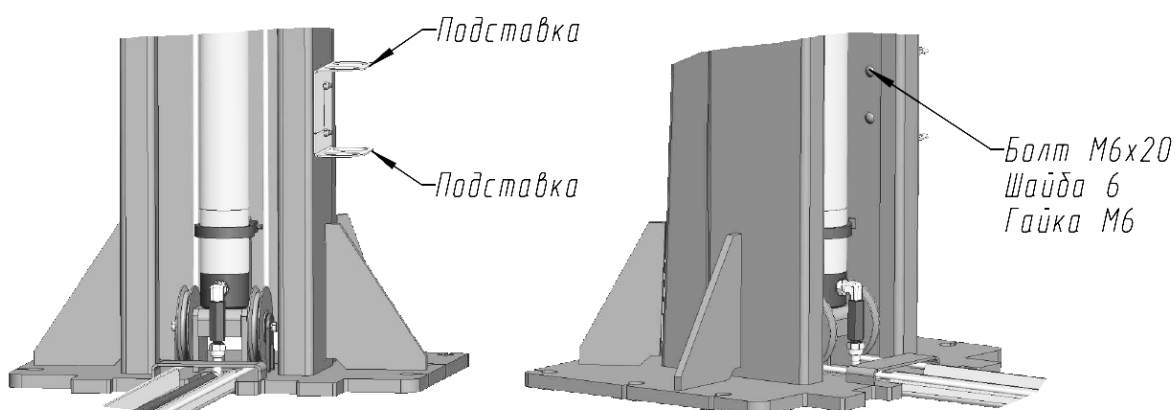
Рисунок 9 - Установка подставок
